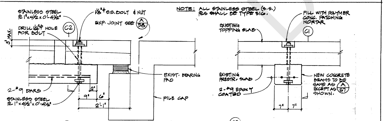
C1 SECTION C 57
