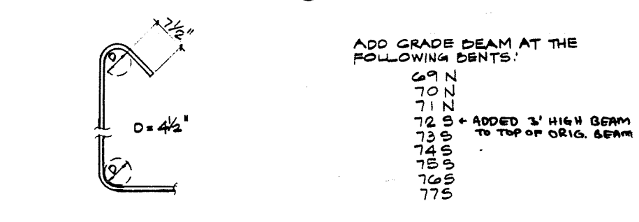
B4 TYP. STIRRUP BENDS
