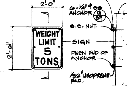
ELEVATION SECTION SIGN DETAIL N.T.S.
