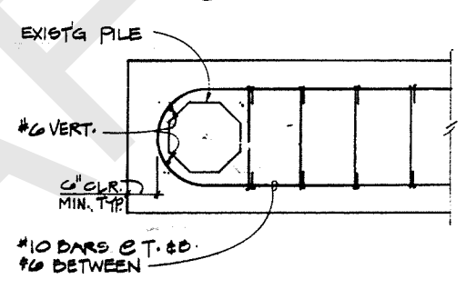
B3 PLAN SECTION
