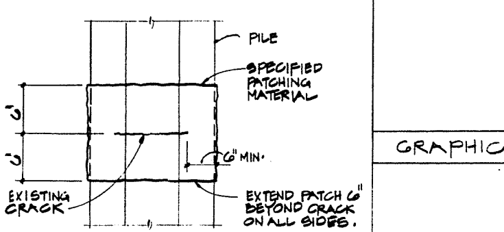
(D) 55 TYPICAL PILE CAP REPAIR
