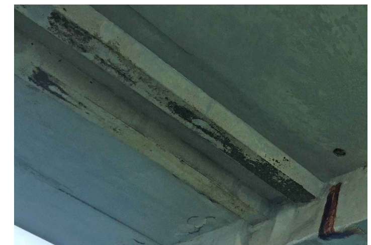
LONGITUDINAL BEAM DAMAGE
