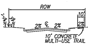
MULTI-USE TRAIL SECTION 3 N.T.S.
