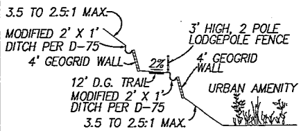
URBAN AMENITY TRAIL SECTION 2 N.T.S.
